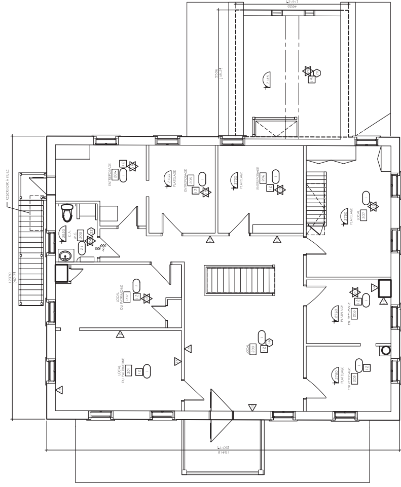
ÉTAGE 1/300 POINTS DE COORDONNÉE
